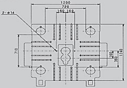
固定盤 FIXED PLATEN
