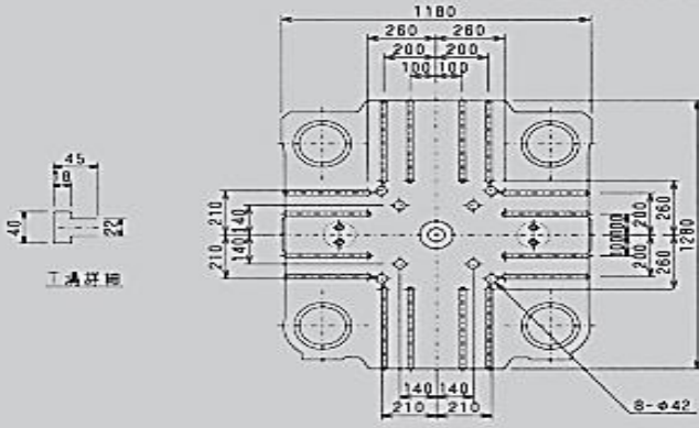
可動盤 MOVABLE PLATEN
