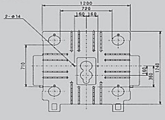
固定盤 FIXED PLATEN
