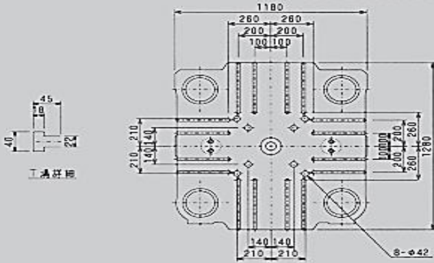
可動盤 MOVABLE PLATEN
