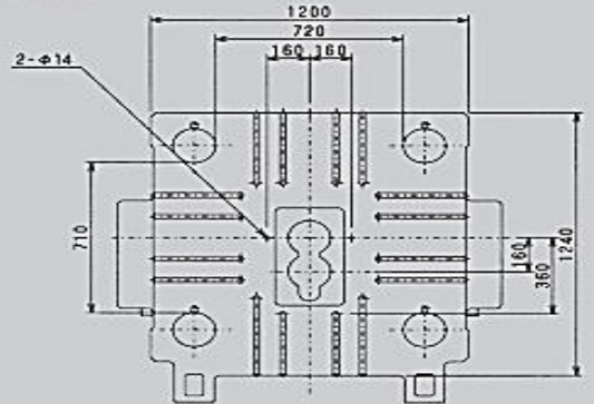
固定盤 FIXED PLATEN
