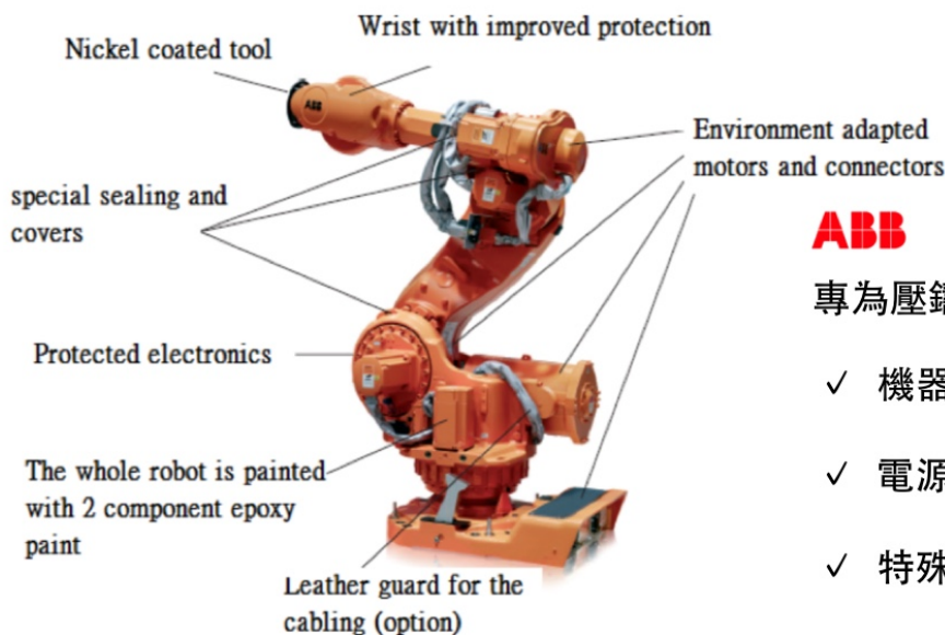
(壓鑄機自動化配置模擬圖)
