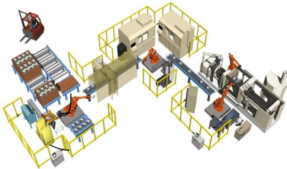
(壓鑄機自動化配置模擬圖)
